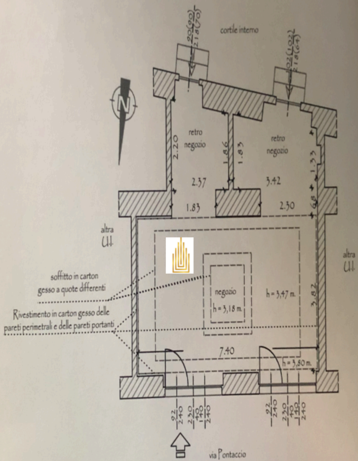
Planimetria stato di fatto
